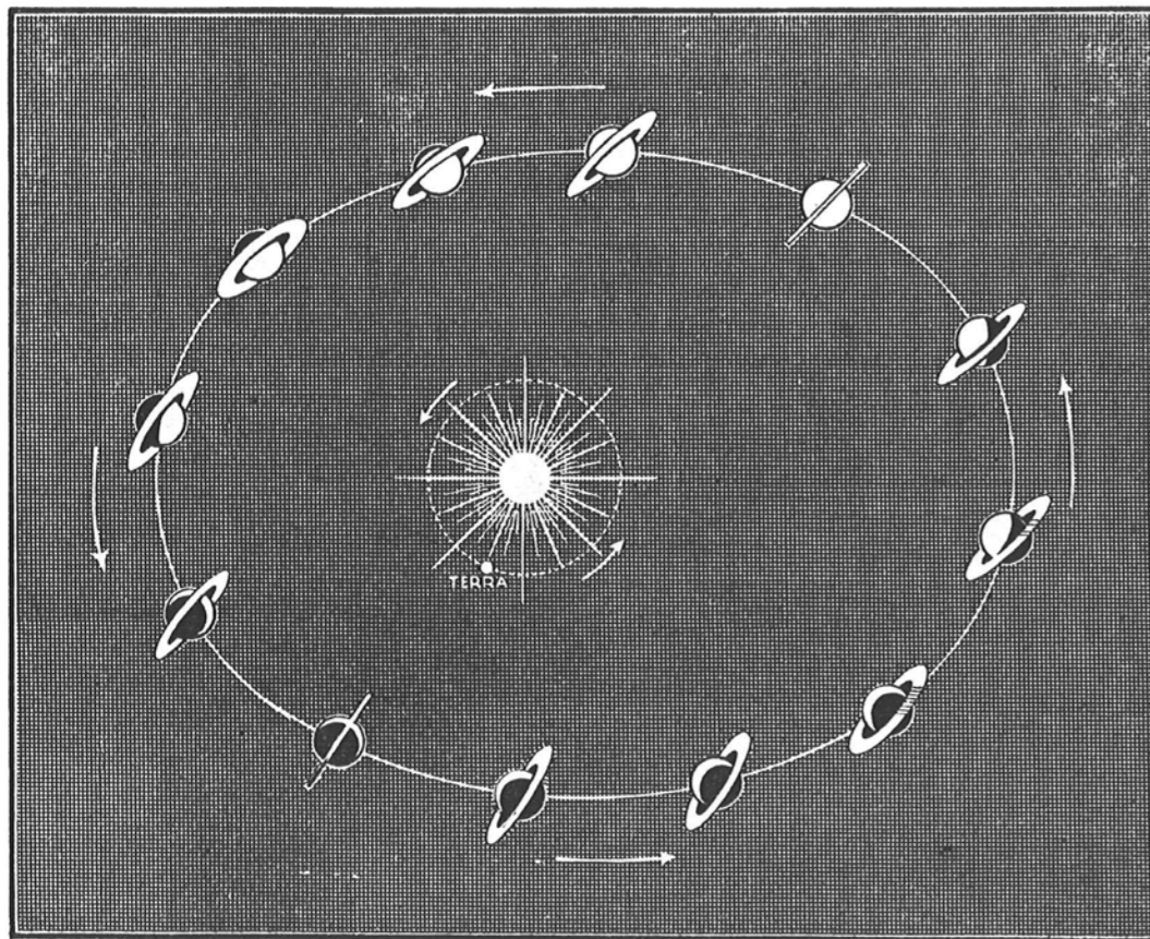
Vari aspetti prospettici del pianeta Saturno osservato da un punto in basso, a sinistra, fuori della sua orbita (pag. 50).
