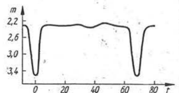
Bedeckungsstern Algol und seine Lichtkurve (m = scheinbare Helligkeit in Größenklas- sen; t = Zeit in Stunden)
